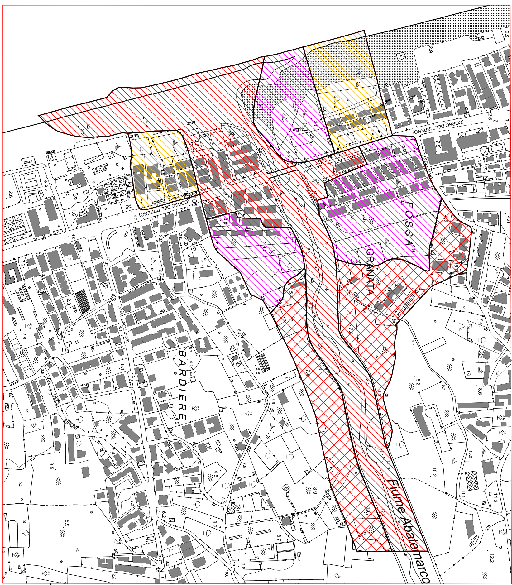
RISCHIO IDRAULICO PERIMETRAZIONE AREE A RISCHIO FIUME ABATEMARCO
